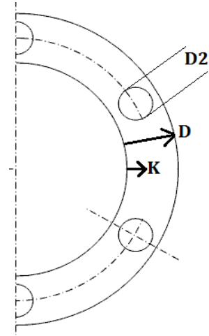
EN-DIN PN 40
